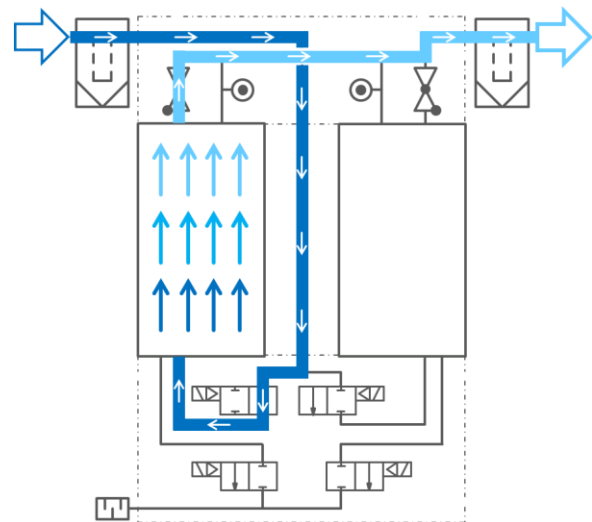
2 Adsorption - Umschaltung
